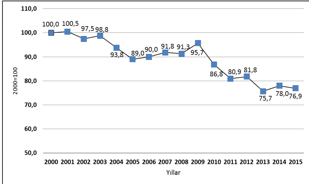
Şekil 2 - Birincil Enerji Yoğunluğu İndeksi Değişimi.
