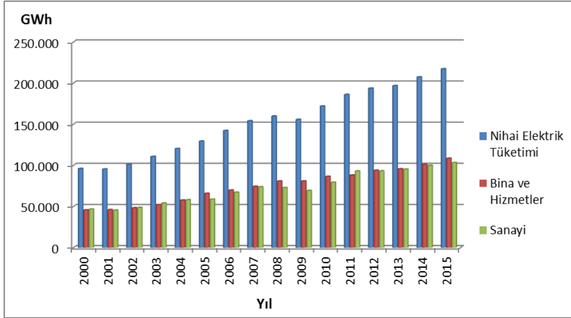
Şekil 8 - Bina ve Hizmetler Sektörü Elektrik Tüketiminin Yıllar İtibariyle Değişimi.
